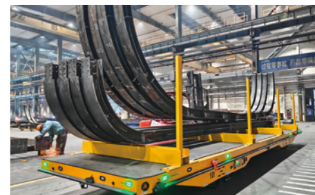
OmniRhino-重载全向运输车(10t)
