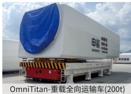
OmniTitan-重载全向运输车(200t)
